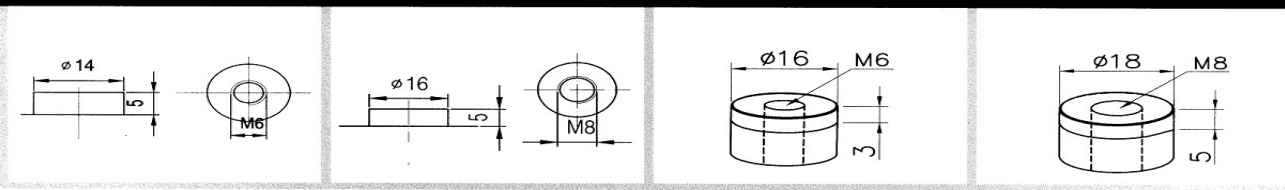
M6/Φ14
